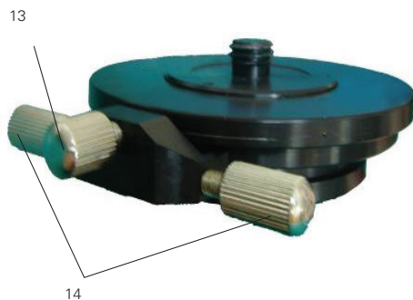
360° Horizontalfeinverstellung
